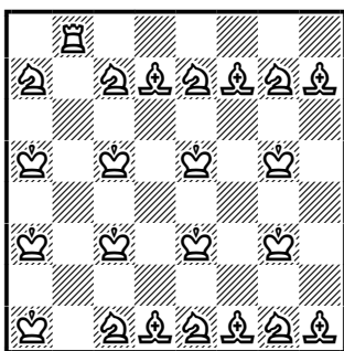
Figuur 1: Optimale configuratie met dreigwaarde 299/224.
