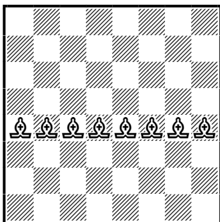
Figuur 2: Configuratie met aanvalswaarde 112.
