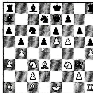
Diagram (Spielmann-Keres)
