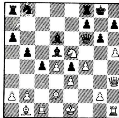
Diagram (Bondarevsky-Smyslov)
