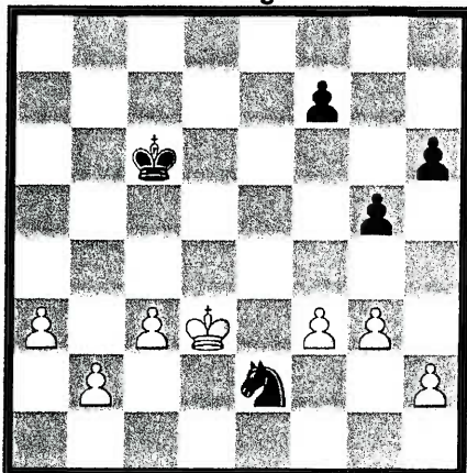
Diagram 8 (eindstand bord 2)
